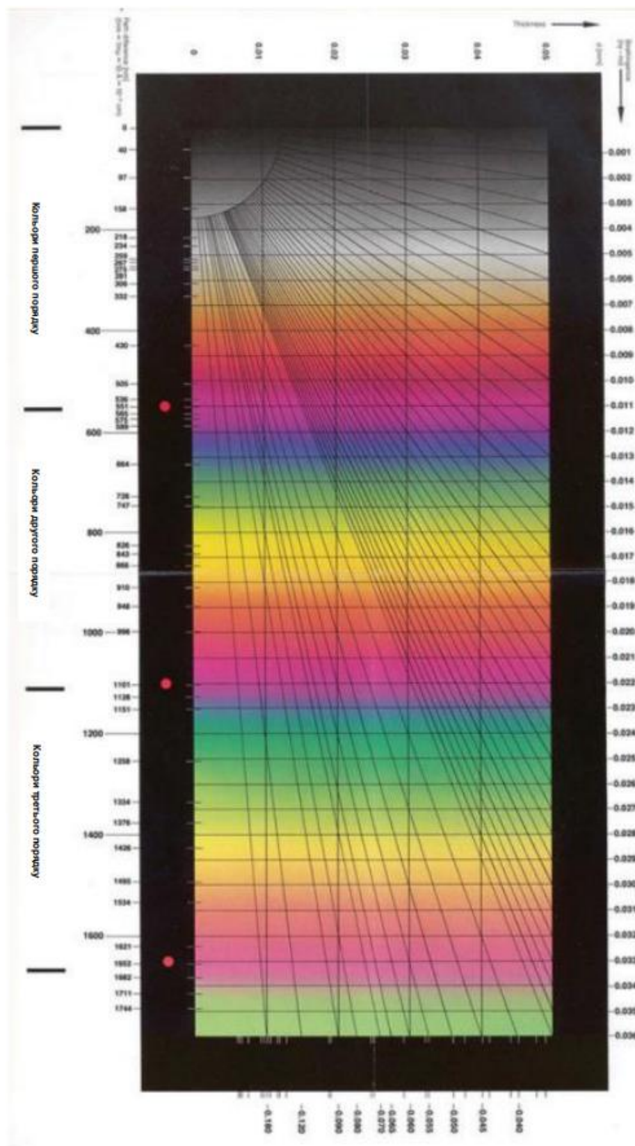
Рисунок В.1 – Діаграма кольорів інтерференції
