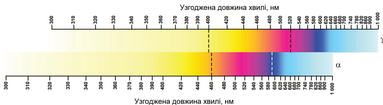
Рисунок С.5 — Кольори дисперсійного забарвлення з центральним стопом для актиноліту в рідині з ПЗ 1,630
