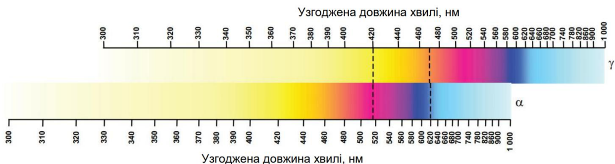
Рисунок С.2 — Кольори дисперсійного забарвлення з центральним стопом для амоситу в рідині з ПЗ 1,680
