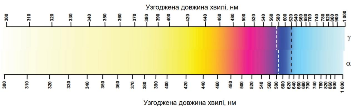
Рисунок С.2 — Кольори дисперсійного забарвлення з центральним стопом для амоситу в рідині з ПЗ 1,680
