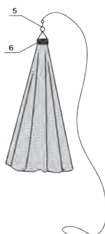
Рис. 3.27. Сіть «Парашут» або кастингова сітка: 1 – центральний тяговий шнур; 2 – стропи; 3 – полотно сітки; 4 – вантажний шнур; 5 – вертлюг; 6 – втулка
